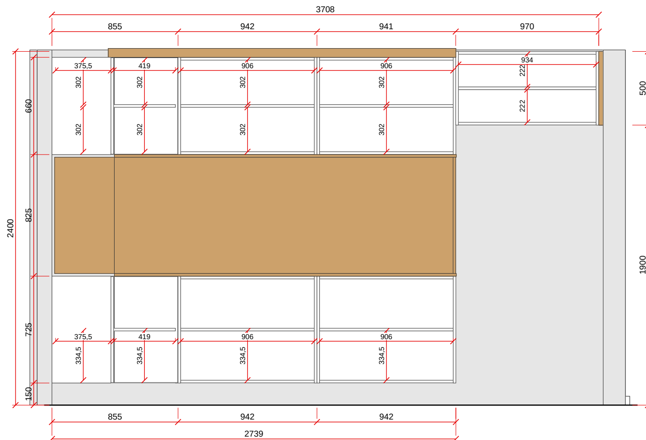
VISTA C - ESC. 1:25
