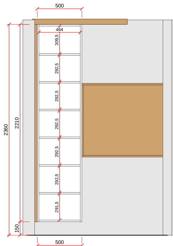
VISTA D - ESC. 1:25
